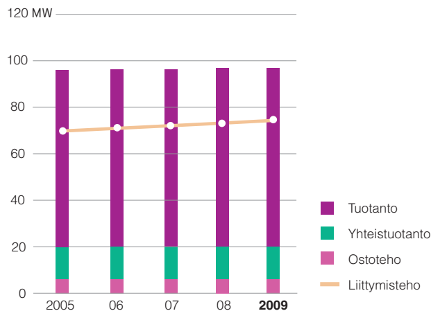
Kaukolämmön yhteistuotanto-, tuotanto-, osto- ja liittymisteho
